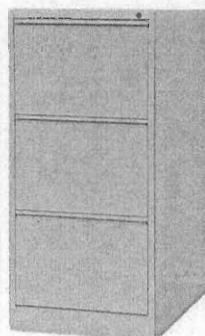
B4-3S S-Handle 462W X 620D X 1062H
